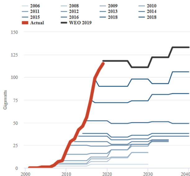
Abbildung 52: IEA-Prognosen seit 2006 und tatsächliche Entwicklung des globalen jährlichen PV-Zubaus [Carb]
