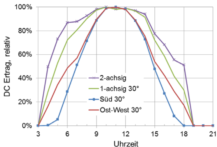
Abbildung 53: Stromertragsprofile von PV-Anlagen in verschiedenen Montagevarianten, berechnet mit der Software PVsol für einen überwiegend klaren Julitag am Standort Freiburg
