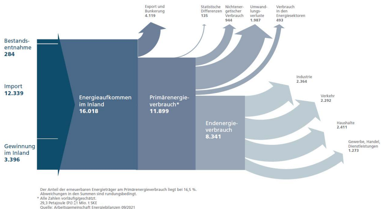
Abbildung 45: Energieflussbild 2020 für Deutschland, Angaben in Petajoule [AGEB2]
