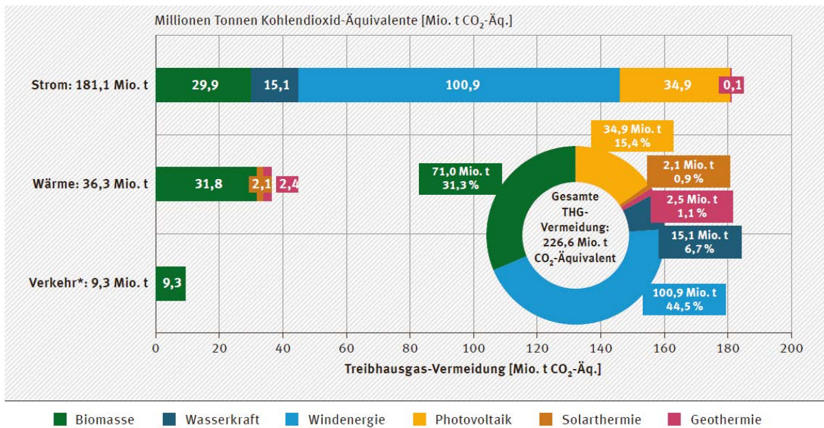
Abbildung 43: Vermiedene Treibhausgasemissionen durch die Nutzung erneuerbarer Energien im Jahr 2020 [UBA1]
