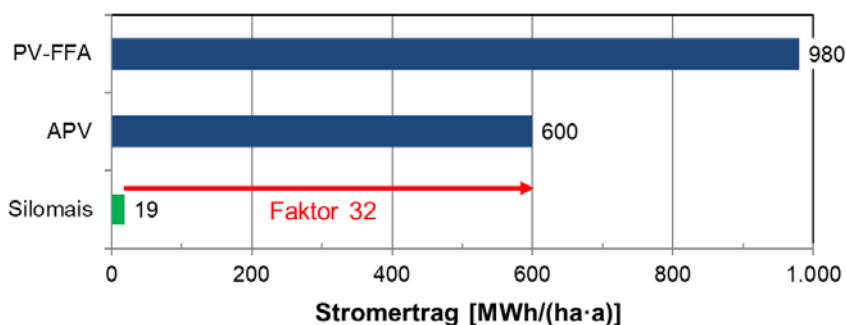
Abbildung 35: Stromerträge von PV-Kraftwerken und Silomais pro Hektar eingesetzter Fläche
