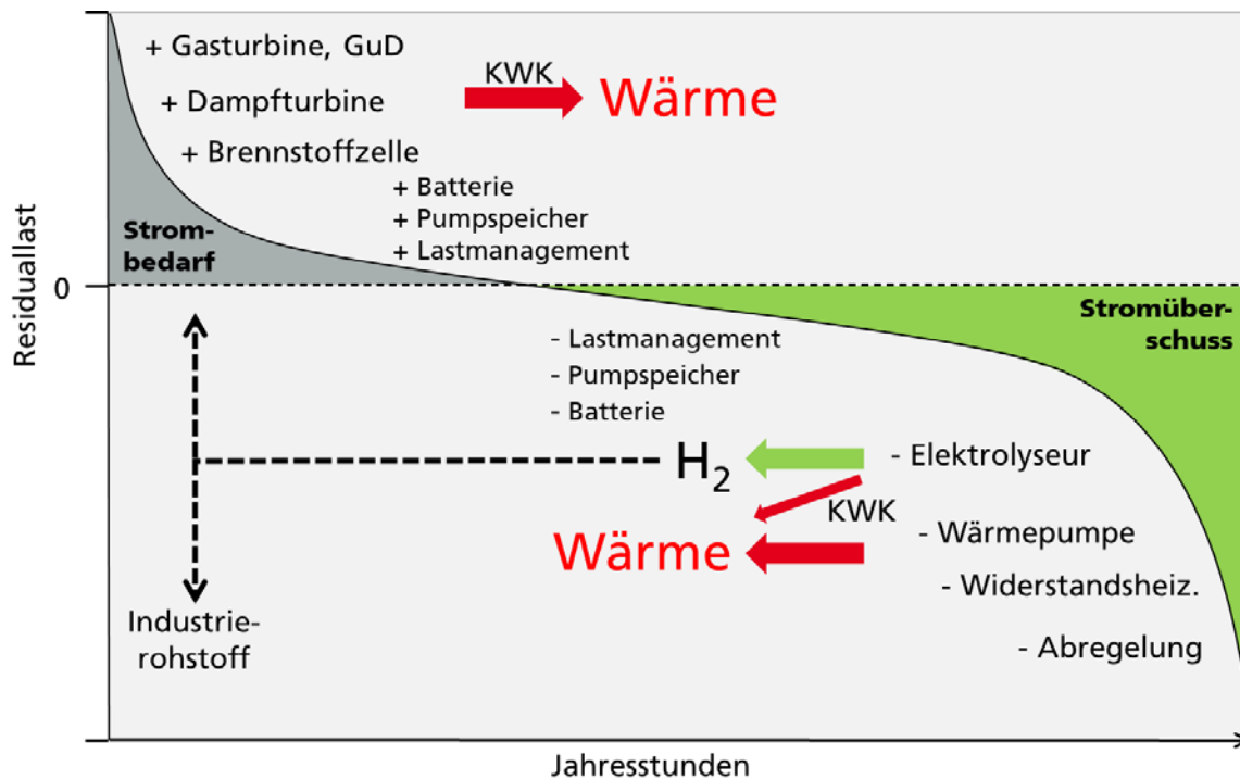
Abbildung 50: Schematische Darstellung einer Residuallastkurve für Deutschland bei Stromversorgung mit 100 % EE, mit Erzeugern (+) und Lasten (-)
