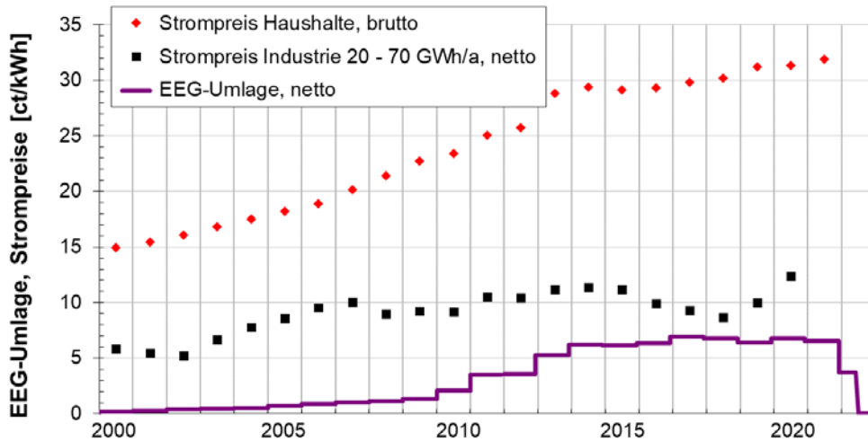
Abbildung 15: Entwicklung von Bruttostrompreisen für Haushalte, von Nettostrompreisen für industrielle Großabnehmer und Entwicklung der EEG-Umlage, Daten aus [BMWK1]
