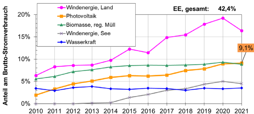
Abbildung 3: Entwicklung des Anteils Erneuerbarer Energien am Bruttostromverbrauch in Deutschland, Daten aus [BMWK1], [BDEW3]
