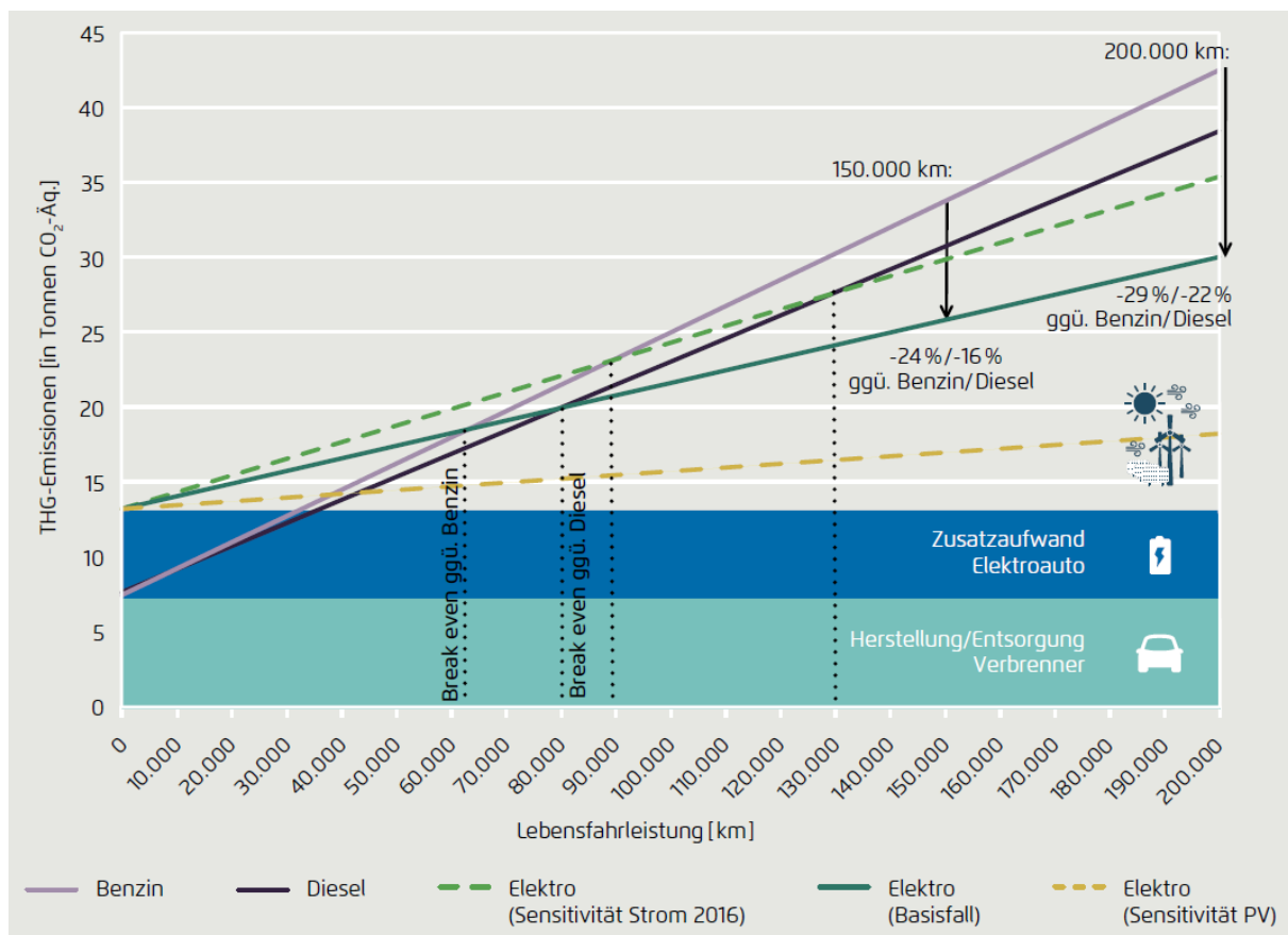
Abbildung 56: Treibhausgasemissionen von heutigen Fahrzeugen der Kompaktklasse in Abhängigkeit von der Fahrleistung [AGORA1]
