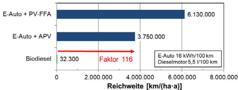
Abbildung 34: Reichweiten von Elektro- und Biodiesel-Fahrzeugen pro Hektar eingesetzter Fläche
