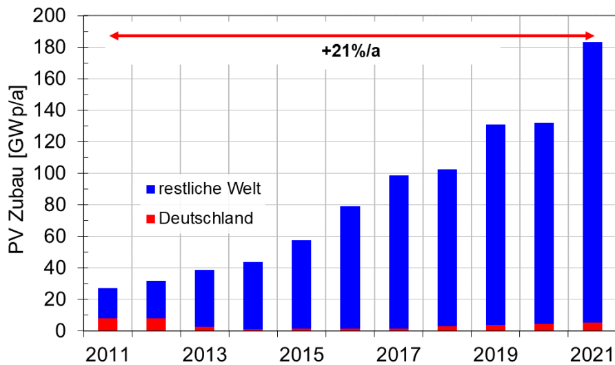
Abbildung 44: Entwicklung des jährlichen PV-Zubaus für Deutschland und die restliche Welt, Zahlen von IHS, Solar Power Europe, Bloomberg NEF.
