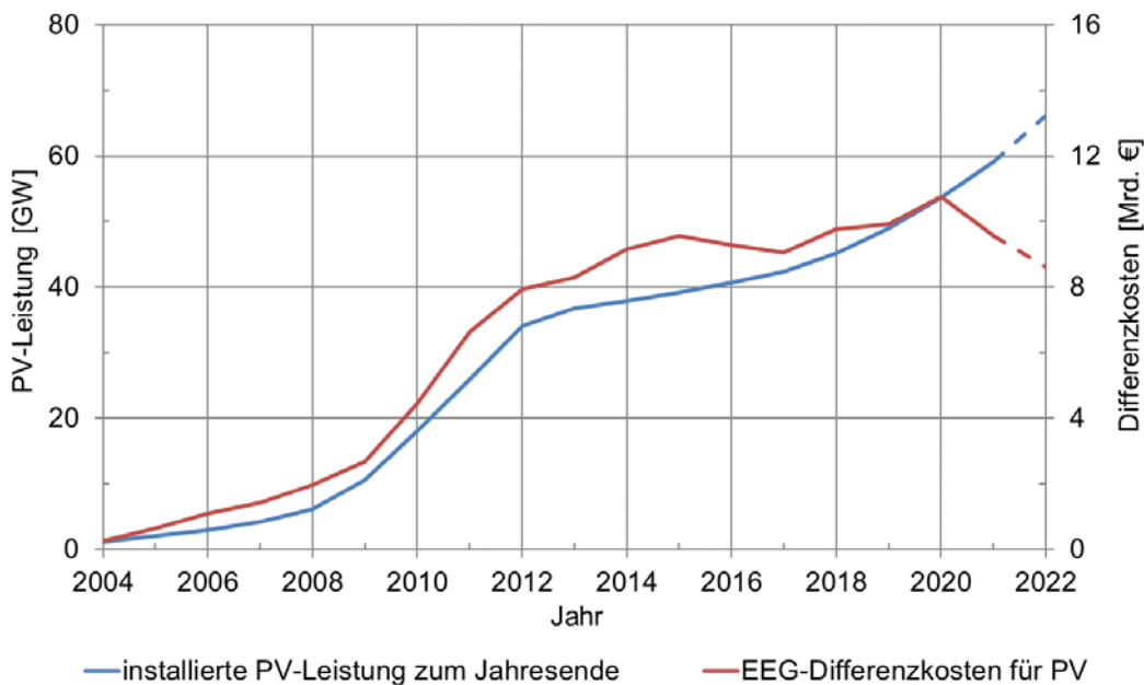
Abbildung 10: PV-Ausbau und Differenzkosten, Daten aus [BMWK1], [BMWK3]
