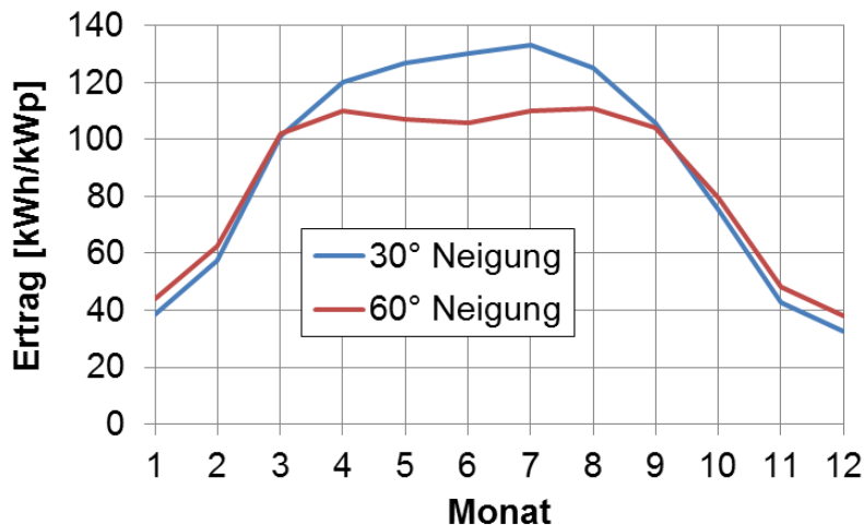
Abbildung 54: Rechenbeispiel für den spezifischen Monatsertrag einer PV-Anlage am Standort Freiburg für südorientierte Module mit 30° Neigung (max. Jahresertrag) und 60° Neigung
